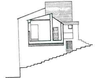
FIANCO
