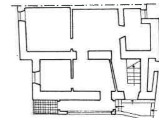
PIANTA PIANO TERZA
