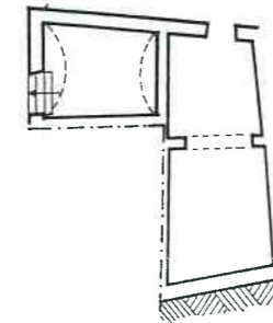
PIANTA FONDI
