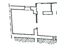
PIANTA PIANO SOTTOSTRADA
