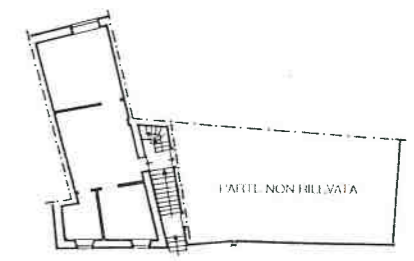
PIANTA MEZZO PIANO
