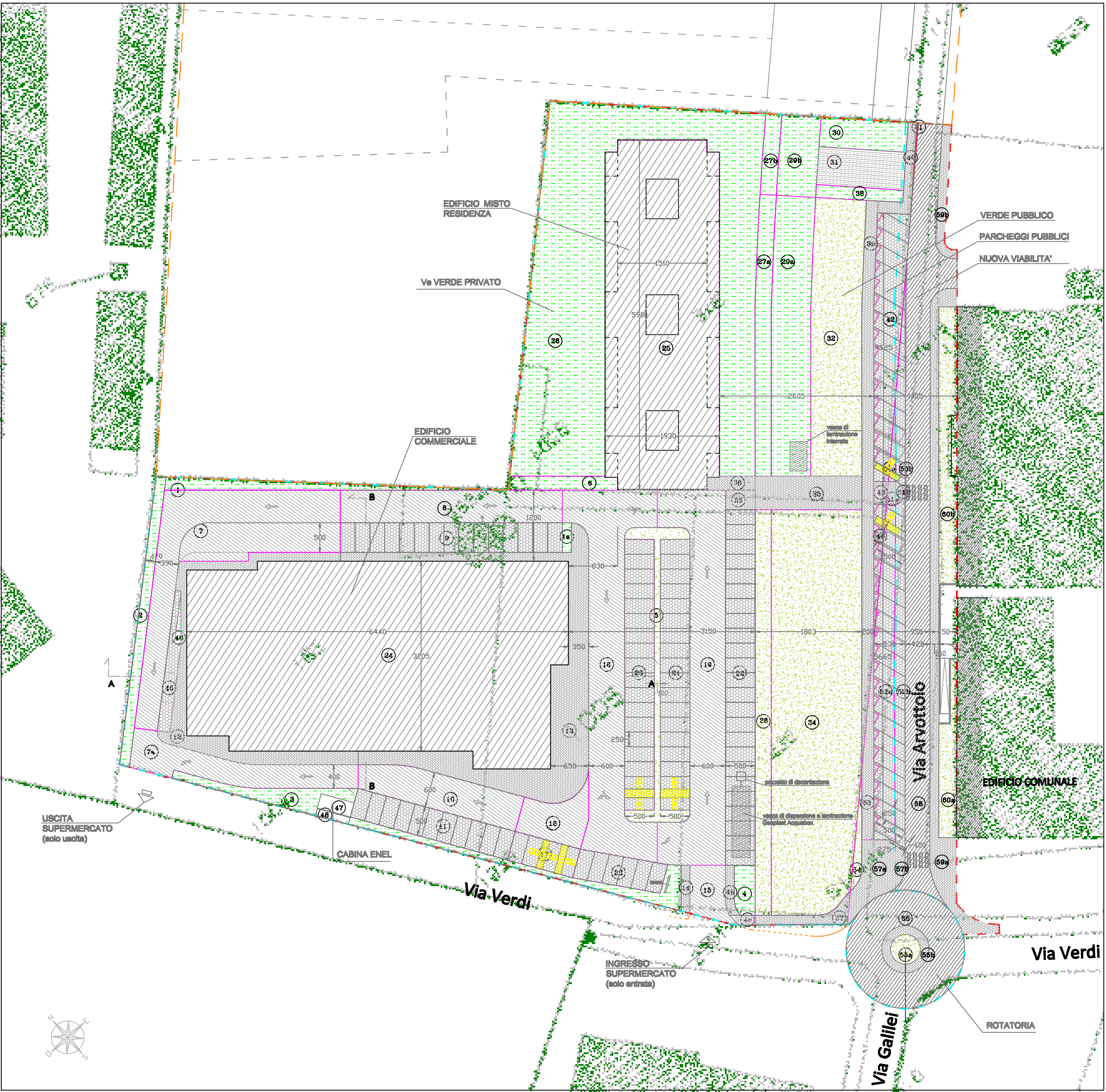
SOU - Planimetria d'insieme
