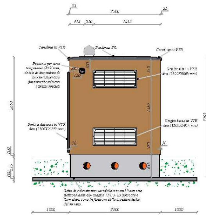
PROSPETTO DX
