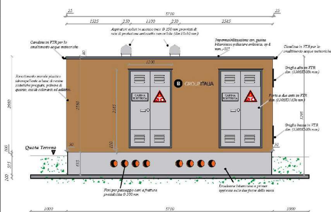
PROSPETTO ANTERIORE
